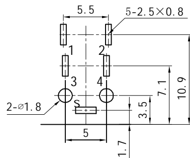
PCB板安装孔图
